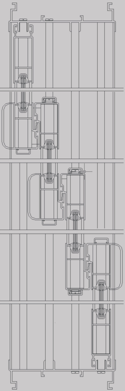
MECAL PLUS 25 Puerta corrediza cuatro hojas cuatro guías
