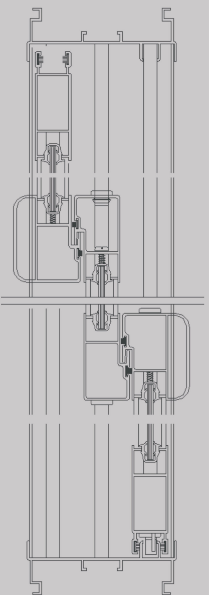
MECAL PLUS 25 Puerta corrediza tres hojas tres guías
